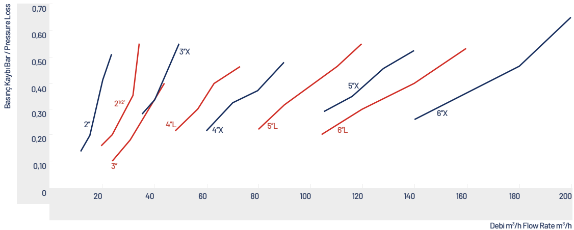
Hidrosiklon Basınç Kaybı Grafiği / Pressure Loss Graph of Hydroclone
